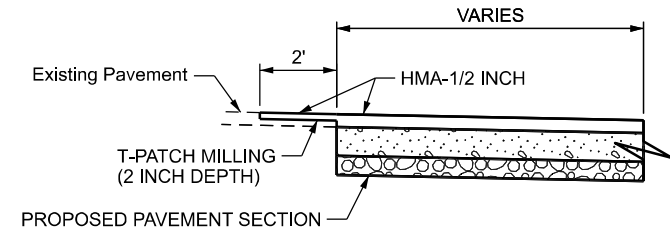
TRANSVERSE T-PATCH SECTION N.T.S.
