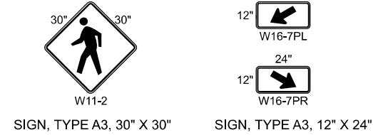
SIGN FACE DETAILS N.T.S.
