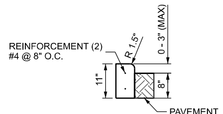
CURB, TYPE P, MODIFIED N.T.S.
