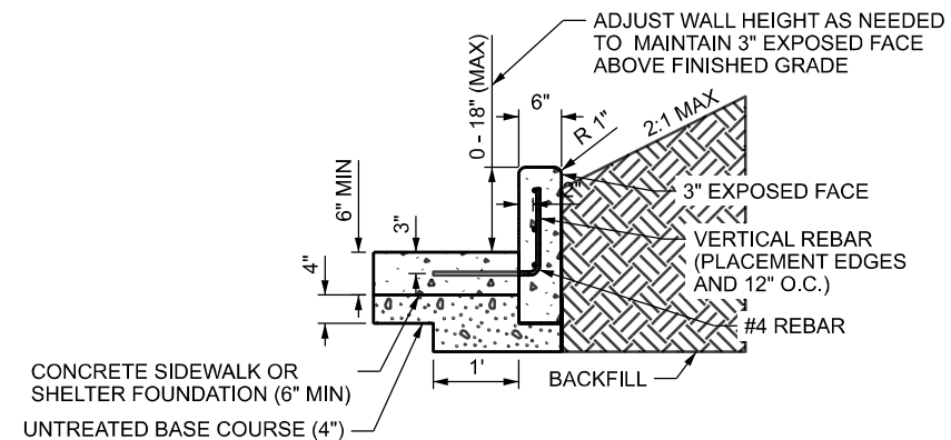
CONCRETE CURB WALL N.T.S.
